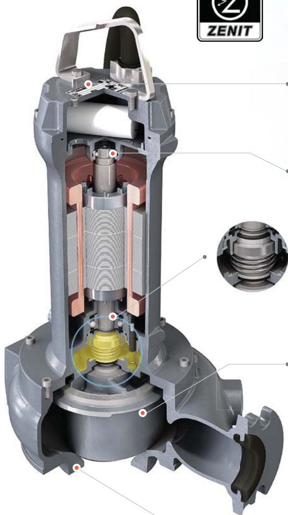
DGG Крыльчатка VORTEX
